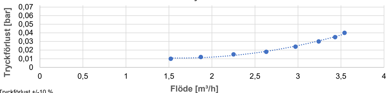
Visades T40F Tryckförlustkurva
